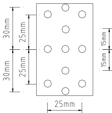
RL ronde gaten
